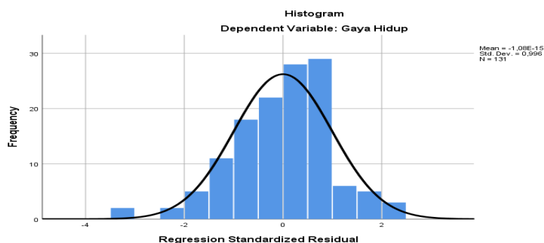
Gambar 1 Grafik Histogram Gaya Hidup
