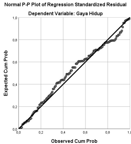
Gambar 2 Grafik Normal P-Plot Gaya Hidup
