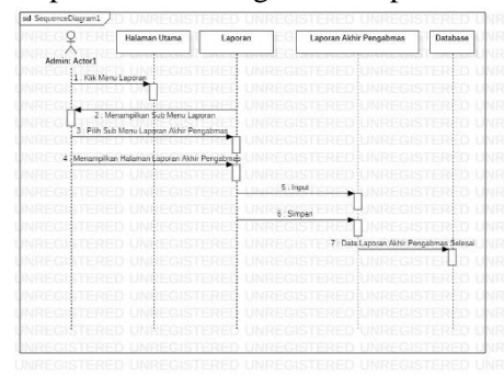
Gambar 41 Sequence Diagram Laporan Akhir Pengabmas
